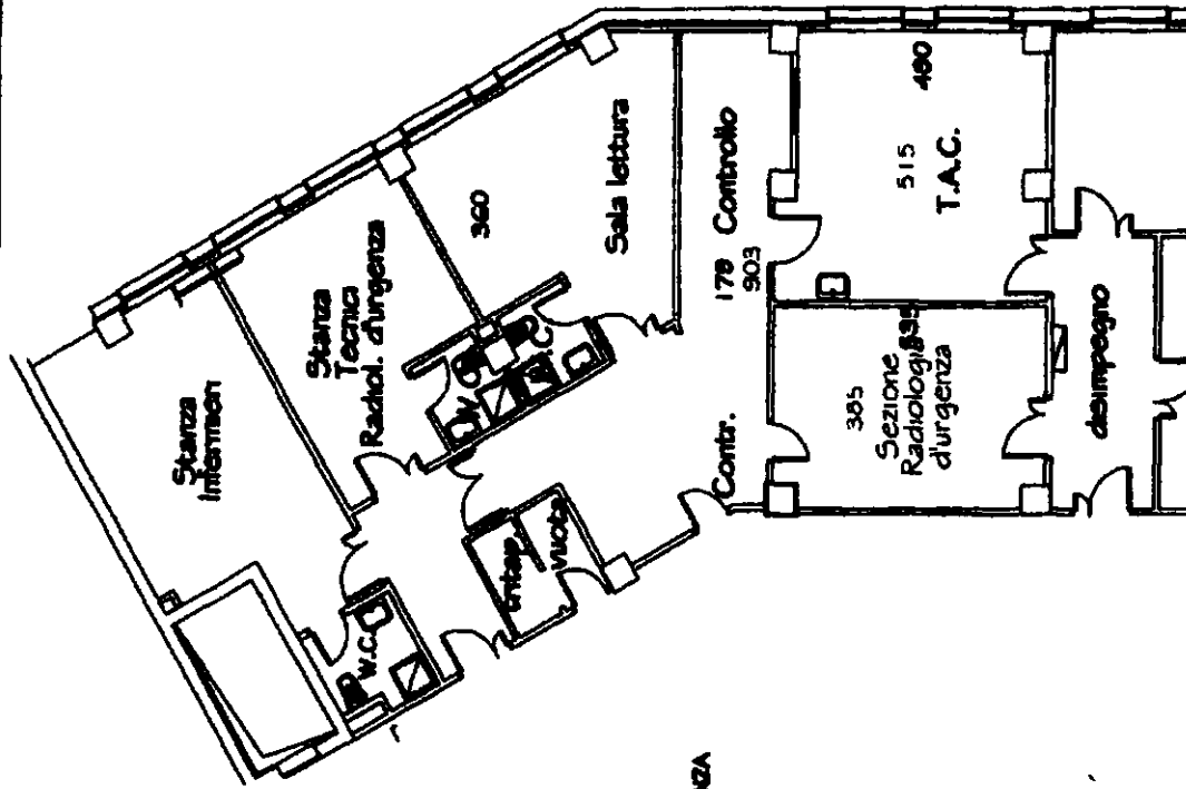
PARTICOLARE DEI LOCALI RADIOLOGIA D'URGENZA
